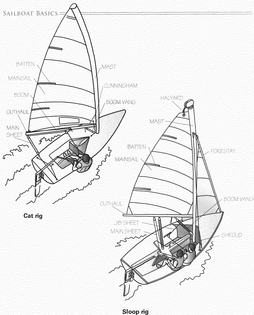
Sloop rig
