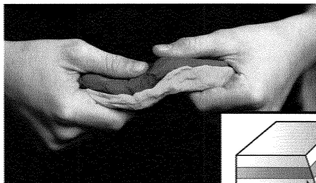
Faults
