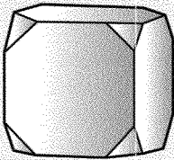
Galena
