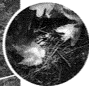
LITTER LAYER
