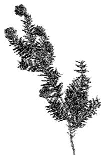
Hemlock
