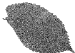
Elm
