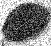
Simple
