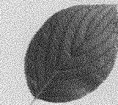
Smooth edge
